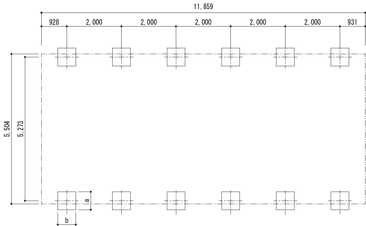
■基礎配置図
